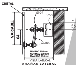
DETALLE DE SUJECCIÓN A ESTRUCTURA POR MEDIO DE CANALES
