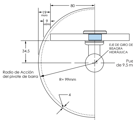
LA PUERTA GIRA DESCENTRADA
