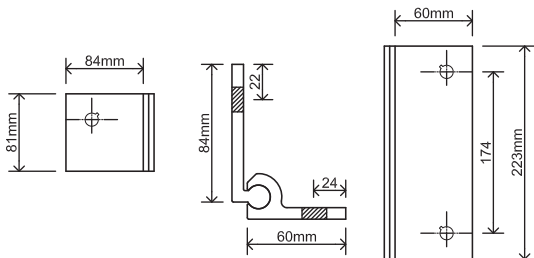
MEDIDAS DE ANGULO ARTICULADO LARGO DE ALUMINIO PARA PUERTA.
