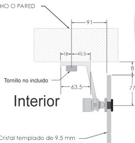
Techo, piso o pared Araña tienda de aluminio de 2 brazos [6162]
