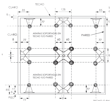
Techo, piso o pared Araña tienda de aluminio de 2 brazos [6162]
