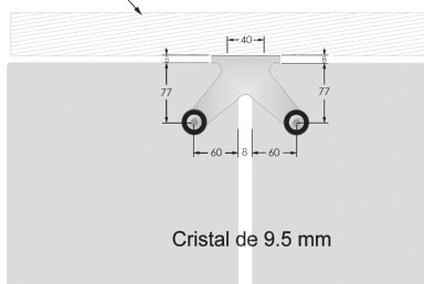
Techo, piso o pared Araña tienda de aluminio de 2 brazos [6162]
