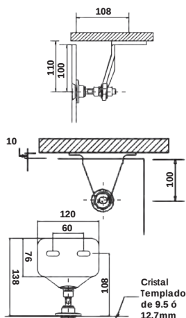
DETALLE DE SUJECCIÓN A TECHO Y A MURO
