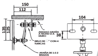
DETALLE DE SUJECCIÓN A ESTRUCTURA POR MEDIO DE CANALES
