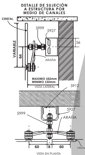
Araña estructural de 128mm con conector cojín
