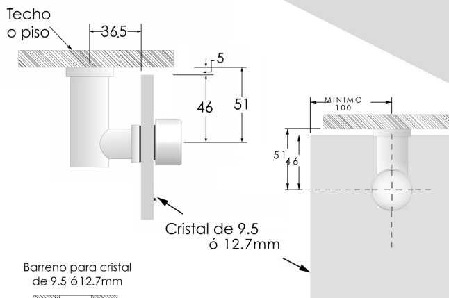
VISTA LATERAL
