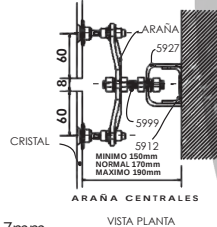
VISTA PLANTA
