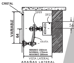
ARAÑAS LATERAL
