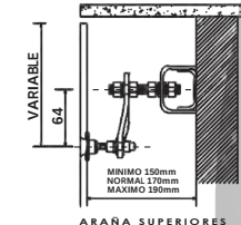
ARAÑA SUPERIORES
