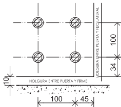
DISTANCIA DE BARRENADO DE CANTOS DE CRISTAL A CENTRO DE BARRENO PARA PIVOTE JUEGO A CERRAMIENTO
