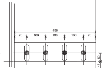
HOLGURA ENTRE FIRME Y COSTILLA
