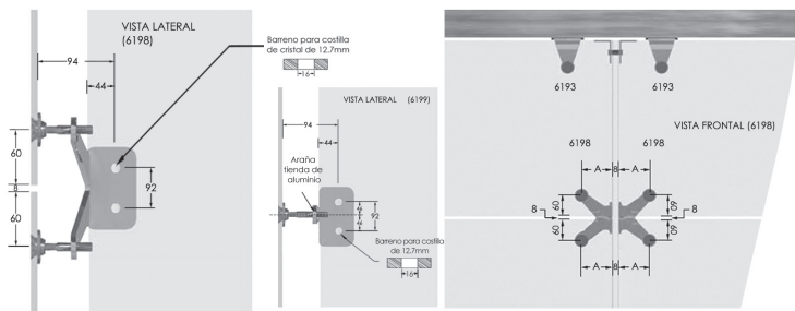
DIBUJO DE BARRENADO DE COSTILLAS PARA ARAÑA TIENDA 128mm A ALETA
