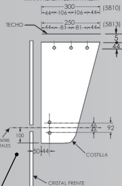
DIBUJO DE BARRENADO DE COSTILLAS PARA ARAÑA TIENDA 128mm A ALETA
