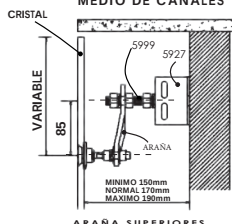
DETALLE DE SUJECIÓN A ESTRUCTURA POR MEDIO DE CANALES
