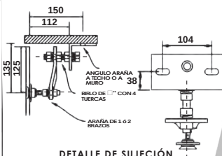
DETALLE DE SUJECIÓN A ESTRUCTURA POR MEDIO DE CANALES
