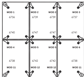
DIAGRAMA DE UBICACIÓN DE ARAÑAS SEGUN MODELO (VISTA POR FUERA)
