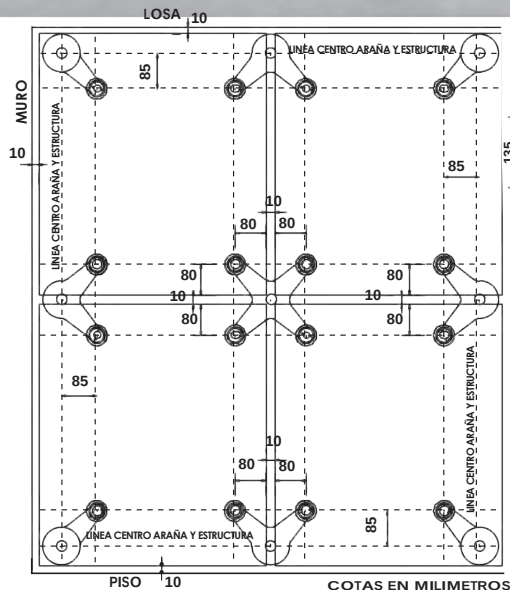
DIAGRAMA DE UBICACIÓN DE ARAÑAS SEGUN MODELO (VISTA POR FUERA)
