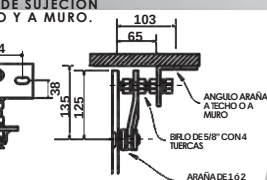
DETALLE DE SUJECIÓN A ESTRUCTURA POR MEDIO DE CANALES
