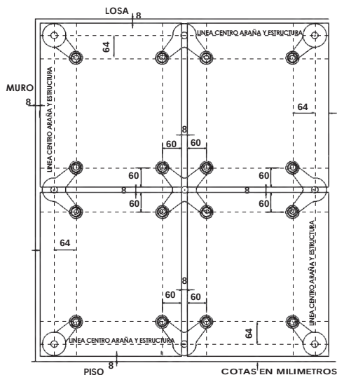
DIAGRAMA DE UBICACIÓN DE ARÁÑAS SEGÚN MODELO (VISTA POR FUERA)
