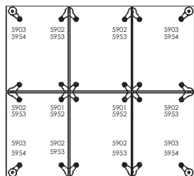
DIAGRAMA DE UBICACIÓN DE ARÁÑAS SEGÚN MODELO (VISTA POR FUERA)
